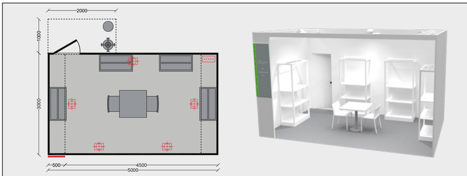
Ripostiglio esterno con apertura porta interna, posizionato su lato sinistro dello stand / External storage room with internal door opening, positioned on the left side of the stand
